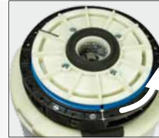
Fig. 6 Svitare la pietra superiore in senso antiorario.
