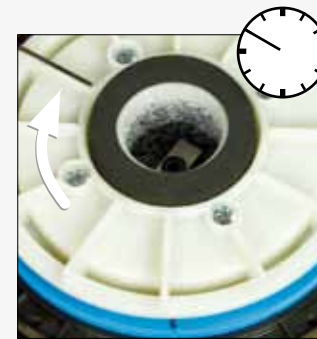
Fig. 8 Avvitando assicurarsi che la macina non si metta di storto.
